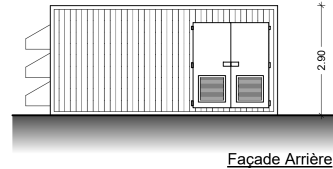
POSTE DE TRANSFORMATION (PT1, PT2 et PT3)
